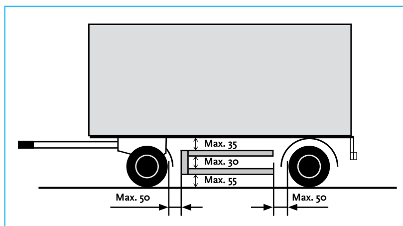
Figuur 1. Zijdelingse afscherming autonome aanhangwagen.
