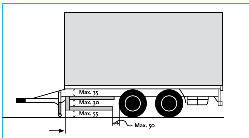
Figuur 2. Zijdelingse afscherming middenaanhangwagens en aanhangwagens met stijve dissel
